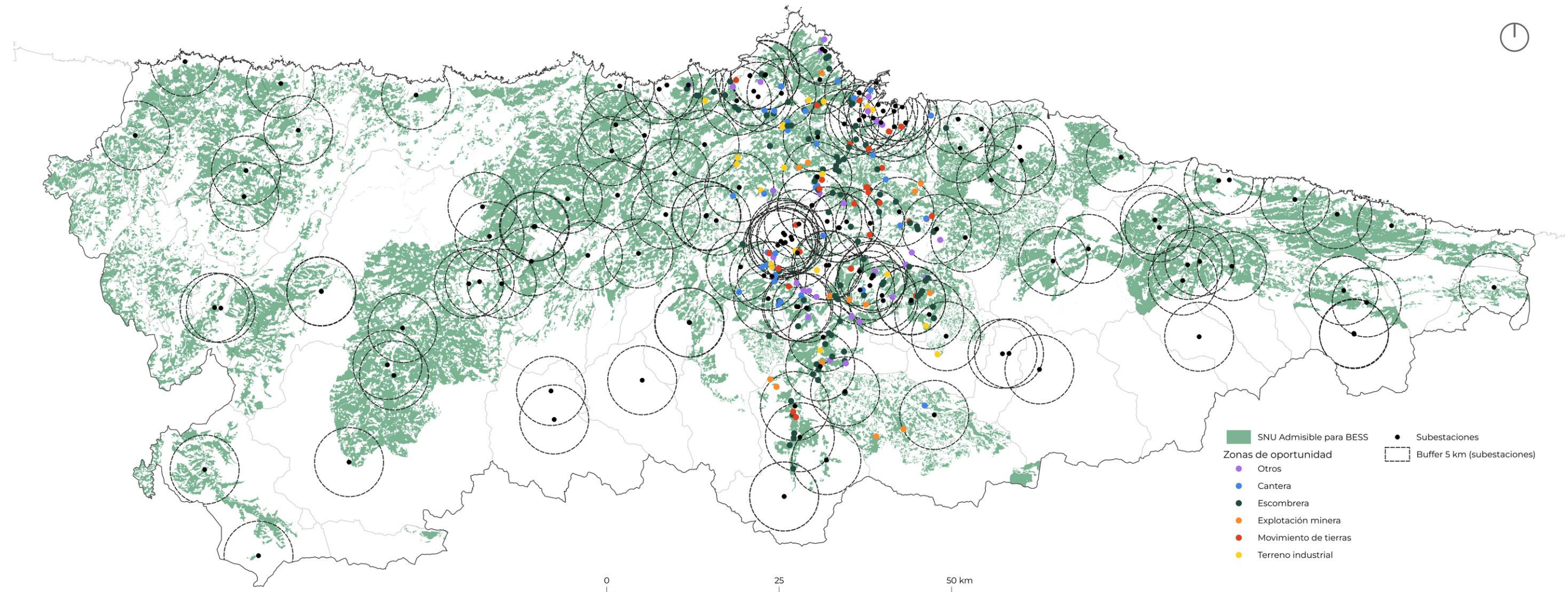
Plano 5. Superposición de subestaciones, radios de 5 km y zonas de oportunidad al SNU admisible para BESS.
