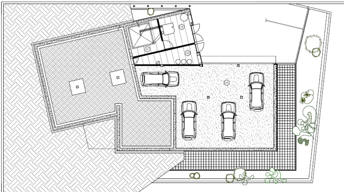
PLANTA SEMISÓTANO INSTALACIONES
