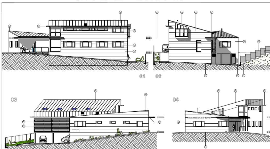
ALZADOS
